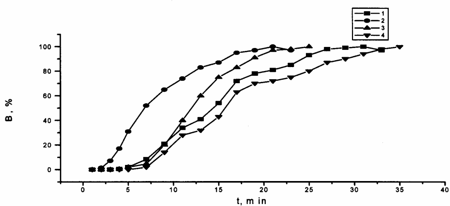
Fig. 2. Variația indicelui de fotoreticulare B în funcție de timp la un conținut diferit de cloranil: 1 - CAMC:OMA (60:40)+10% CHI3+1% ClAn; 2 - CAMC:OMA (60:40)+10% CHI3+2% ClAn; 3 - CAMC:OMA (60:40)+10% CHI3+3% ClAn; 4 - CAMC:OMA (60:40)+10% CHI3+4% ClAn.
